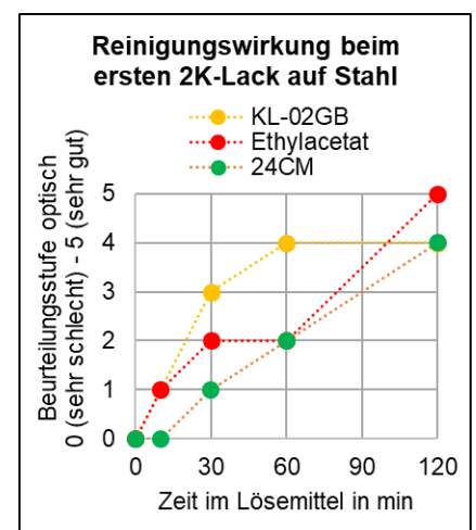
Abbildung 1: Vergleich der Reinigungswirkung
