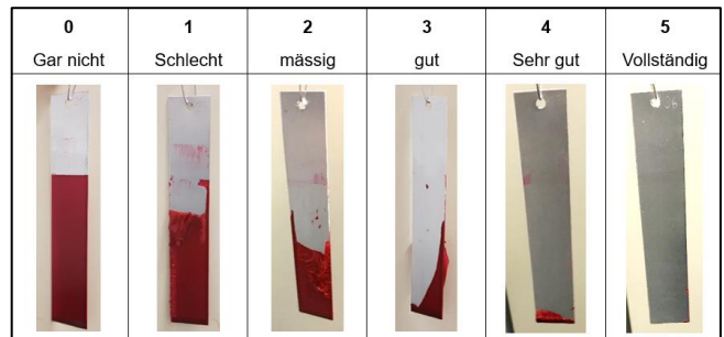
Abbildung 4: Beurteilungsstufen für die optische Beurteilung
